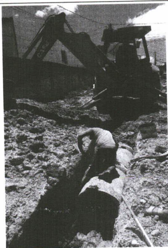
ASSENTAMENTO DE TUBOS DE CONCRETO
