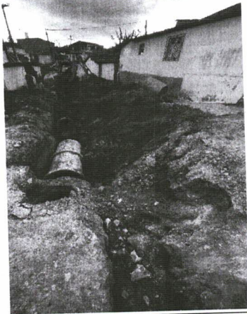
ASSENTAMENTO DE TUBOS DE CONCRETO
