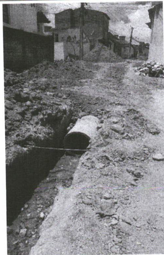
ASSENTAMENTO DE TUBOS DE CONCRETO
